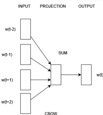
GAMBAR 2. Ilustrasi Arsitektur Word2vec CBOW
