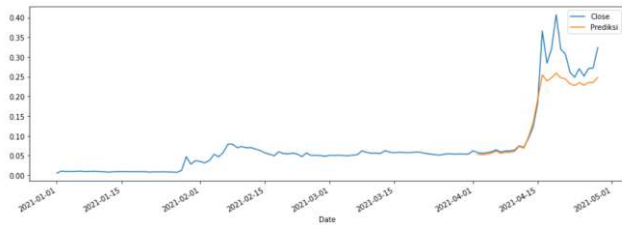
GAMBAR 14. Visualisasi pengujian kedua
