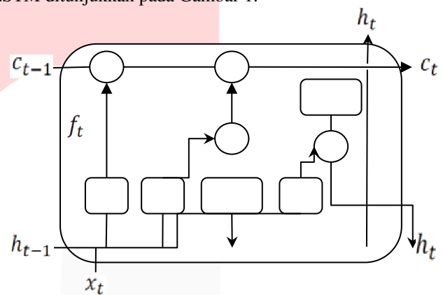
GAMBAR 1. Struktur Unit LSTM
