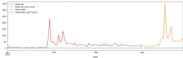
GAMBAR 11. Visualisasi data doge close dan sum score pada pengujian kedua
