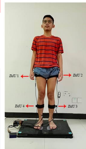
GAMBAR 4.2 Alat ketika digunakan partisipan
