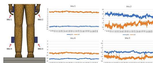
GAMBAR 4.15 Grafik Subjek 1 Mata Terbuka Pitch dan Roll Sensor IMU
