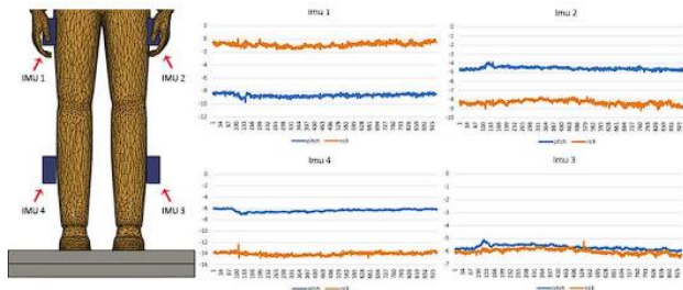
GAMBAR 4.9 Grafik Subjek 1 Pitch dan Roll Sensor IMU
