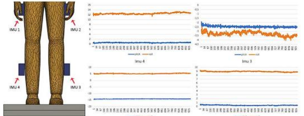
GAMBAR 4.9 Grafik Subjek 1 Pitch dan Roll Sensor IMU
