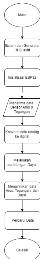
GAMBAR 7 Flowchart Sistem Akuisisi Data
