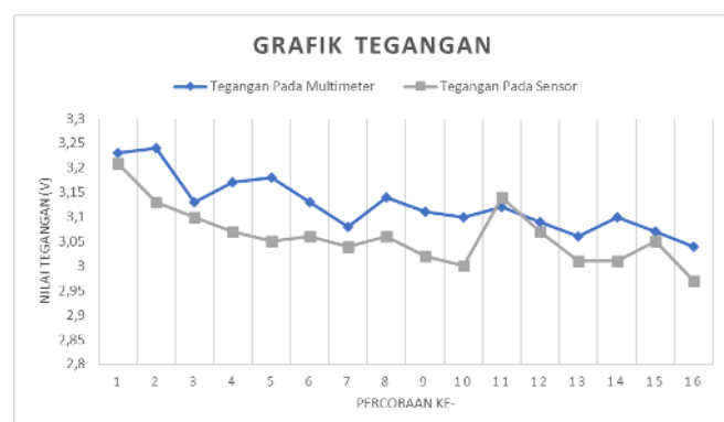
GAMBAR 12 Grafik Sensor Tegangan
