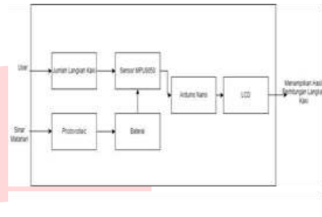
GAMBAR 2. Desain Sistem
