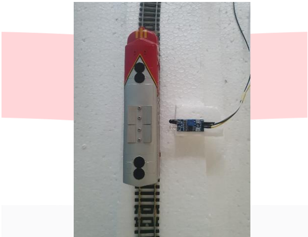
Gambar 4 Sensor IR Mendeteksi Kereta
