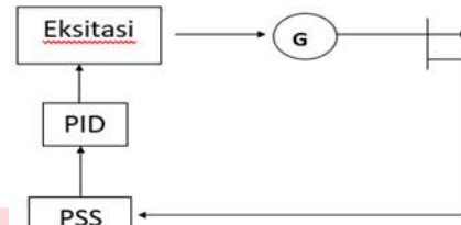
GAMBAR 5 Implementasi PSS PID pada Single Machine
