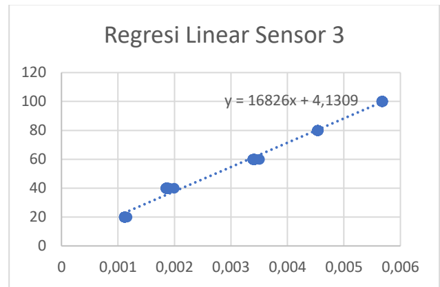
GAMBAR 8 Grafik Sensor 3
