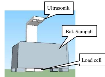
GAMBAR 3 Rancangan desain 3D bak sampah
