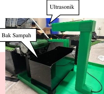
GAMBAR 4 Realisasi prototipe bak sampah (letak ultrasonik)
