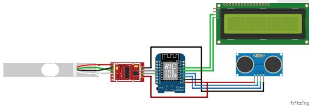
GAMBAR 2 Skema Rangkaian
