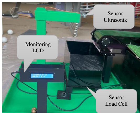
GAMBAR 5 Hasil Integrasi Akhir Sistem
