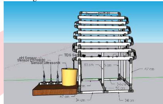
GAMBAR 5 Desain Alat
