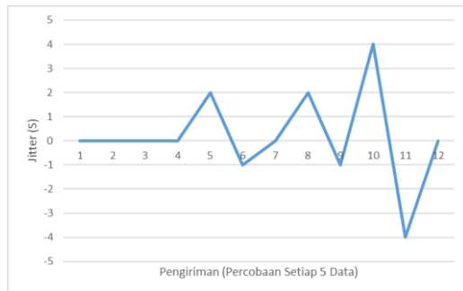
GAMBAR 15 Grafik Pengujian Jitter
