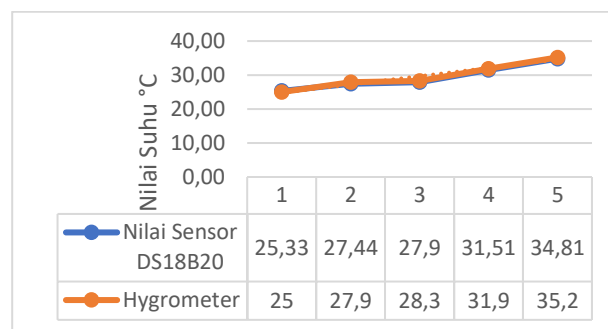
GAMBAR 11 Grafik Hasil Pengujian Sensor DS18B20
