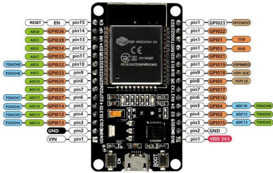
GAMBAR 2. Mikrokontroler ESP32
