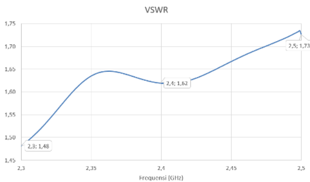
GAMBAR 9 Hasil Pengukuran VSWR HPA
