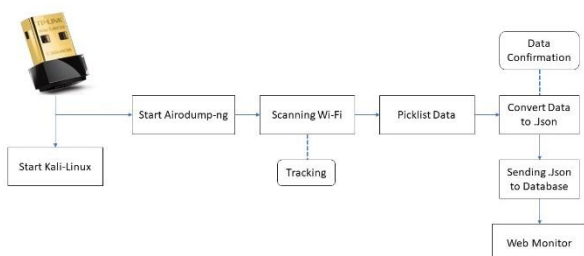
GAMBAR 3.2 Skema infrastruktur deteksi Wi-Fi
