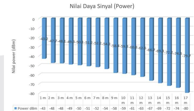
GAMBAR 4.4 Chart sinyal daya (power) Wi-Fi yang diuji
