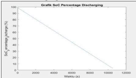
GAMBAR 3.2 Grafik hubungan SoC discharging (%) dengan waktu (s)
