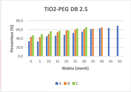
GAMBAR 4. 5 Grafik Persentase Hilangnya Pengotor Debu 2.5 g Pada Permukaan Lapisan TiO 2 -PEG
