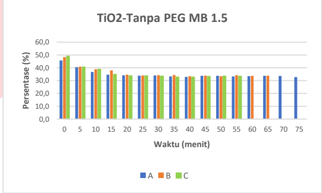
GAMBAR 4. 2 Grafik Persentase Hilangnya Pengotor Methylene Blue 1.5 ml Pada Permukaan Lapisan TiO 2 - Tanpa PEG
