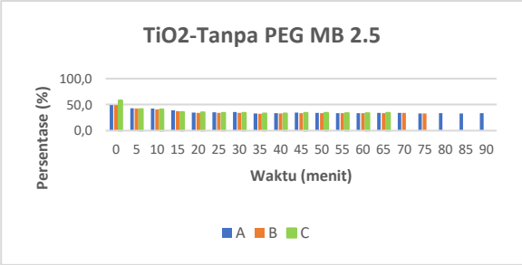
GAMBAR 4. 3 Grafik Persentase Hilangnya Pengotor Methylene Blue 2.5 ml Pada Permukaan Lapisan TiO 2 - Tanpa PEG
