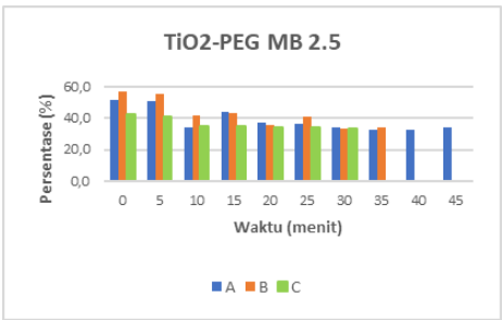
GAMBAR 4. 3 Grafik Persentase Hilangnya Pengotor Methylene Blue 1.5 ml Pada Permukaan Lapisan TiO 2 -PEG
