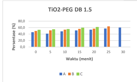
GAMBAR 4. 4 Grafik Persentase Hilangnya Pengotor Debu 1.5 g Pada Permukaan Lapisan TiO 2 - PEG
