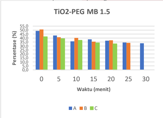
GAMBAR 4. 2 Grafik Persentase Hilangnya Pengotor Methylene Blue 1.5 ml Pada Permukaan Lapisan TiO 2 -PEG
