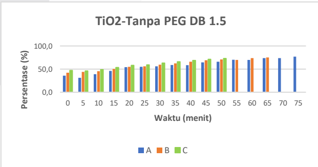
GAMBAR 4. 6 Grafik Persentase Hilangnya Pengotor debu 1.5 g pada lapisan TiO 2 -Tanpa PEG
