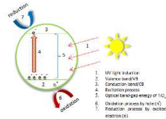
GAMBAR 2.2 Mekanisme Fotokatalis [14]
