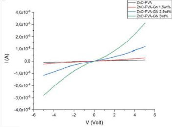
GAMBAR 4. 1. Perbandingan Respon I-V ZnO-PVA dengan ZnO-PVA-Graphene
