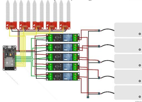
GAMBAR 3.1 Skematik Rangkaian
