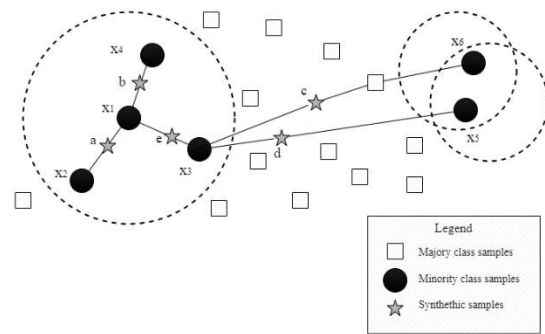
GAMBAR 2. Ilustrasi SMOTE
