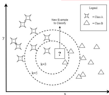
GAMBAR 1. Ilustrasi algoritma K-NN
