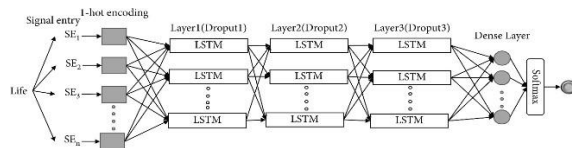
GAMBAR 1 Arsitektur LSTM
