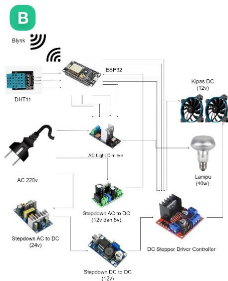
GAMBAR 9 Arsitektur Utama Sistem
