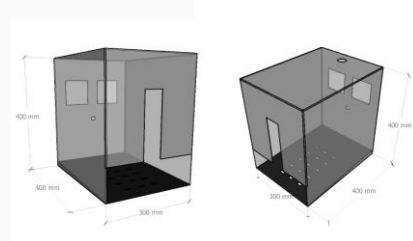
GAMBAR 1 Desain kandang
