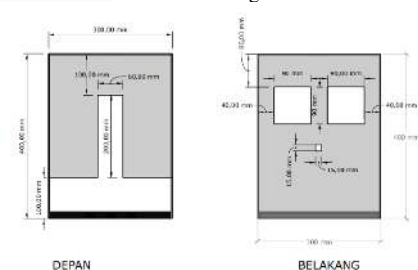
GAMBAR 2 Tampak depan dan belakang
