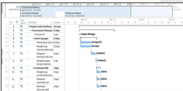
GAMBAR 5 Jadwal Usulan (Kombinasi Fast tracking dan Crashing )
