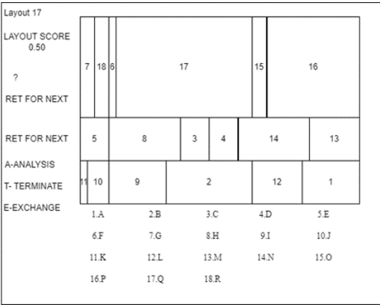
GAMBAR IV. 2 Layout Usulan
