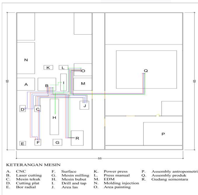
GAMBAR IV.2 Layout Sementara
