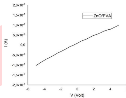
GAMBAR 2. Grafik Respon I-V Nanokomposit ZnO/PVA
