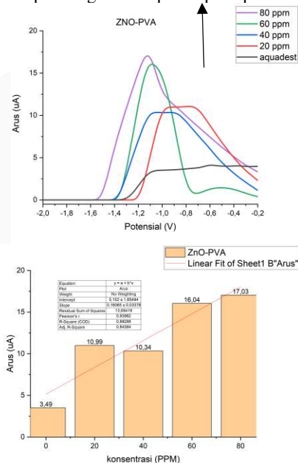
GAMBAR 6. Puncak Respon Pendeteksian SWV dan Fitting Linearitas Respon Keluaran
