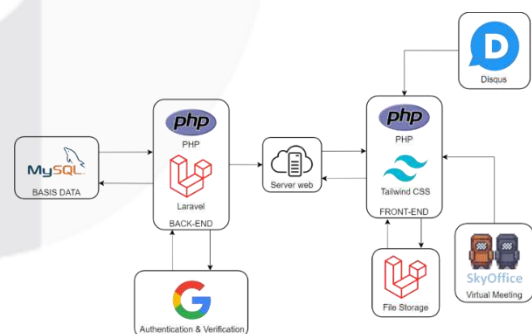
GAMBAR 2 Arsitektur lengkap website aplikasi Fateka
