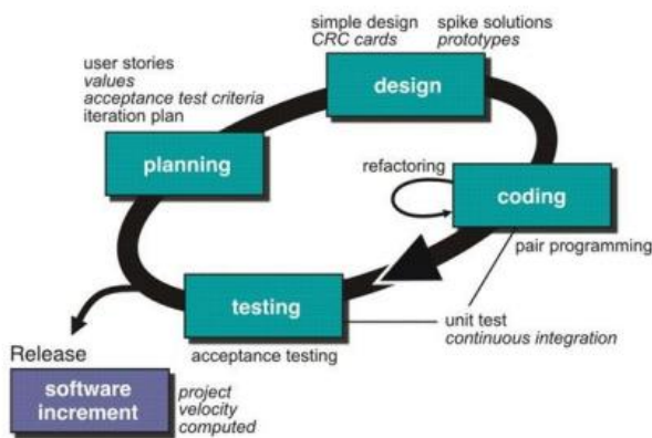
GAMBAR 1 Fase pada Extreme Programming
