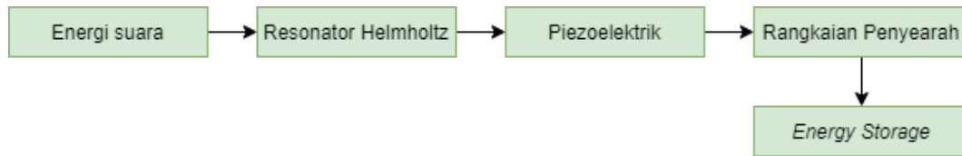
Gambar 3. 1 Diagram Blok Sistem
