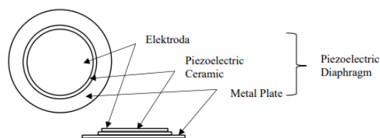
Gambar 2. 1 Susunan Elemen Piezoelektrik[7]
