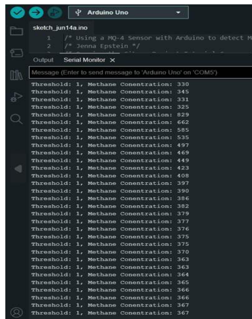
GAMBAR 6 Pengujian sensor konsentrasi gas
