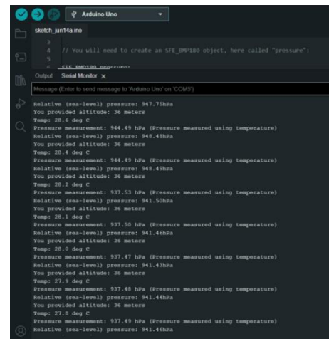
GAMBAR 5 Pengujian sensor tekanan
