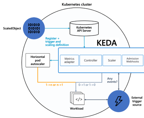
GAMBAR 2 ARSITEKTUR KEDA
