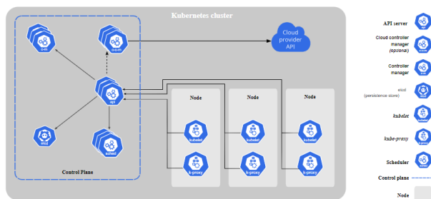
GAMBAR 1 ARSITEKTUR KUBERNETES
