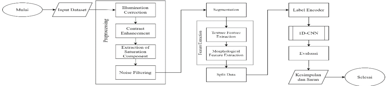
GAMBAR 1. ALUR PEMODELAN
