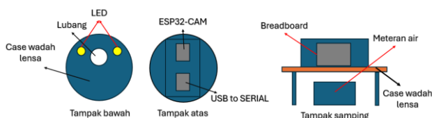
GAMBAR 1. SKETSA PERANGKAT
