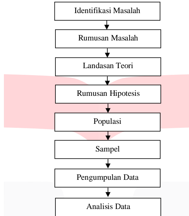
Gambar 1. Tahapan Penelitian
