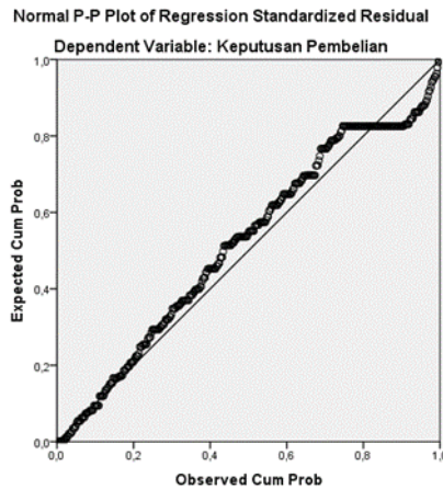
Gambar 3.1 Grafik Uji Normalitas P-Plot
