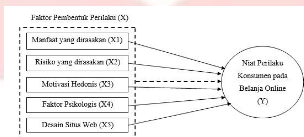
Gambar 2.1 Kerangka Pemikiran
