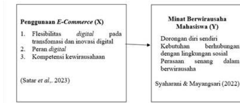
Gambar 1. Kerangka Pemikiran
