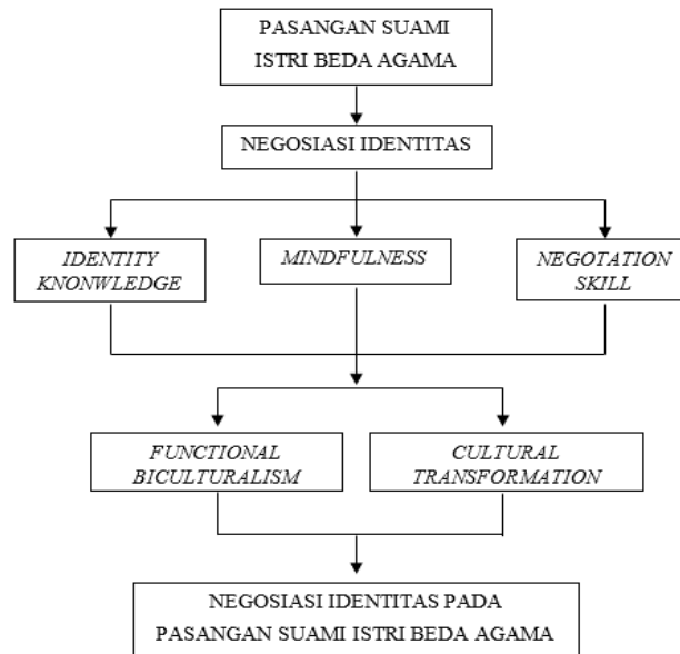
Gambar 2.1 Kerangka Pemikiran
