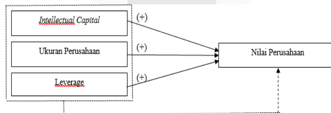
Gambar 1 Kerangka Pemikiran
