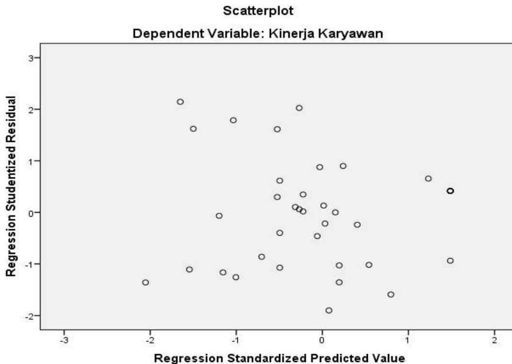
Gambar 3 Uji Heteroskedastisitas
