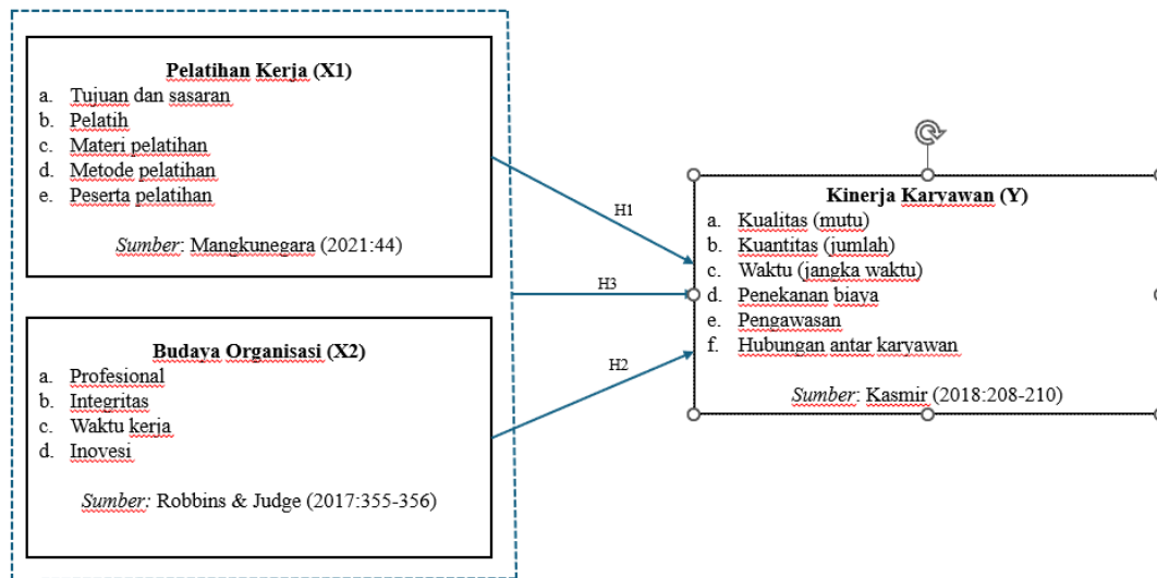
Gambar 1 Kerangka Pemikiran
