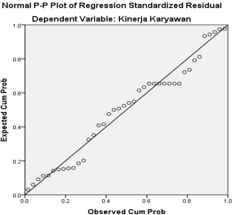
Gambar 2 Uji Normalitas
