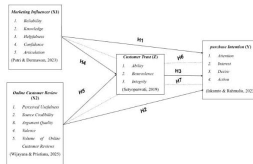
Gambar 2.1 Kerangka Pemikiran
