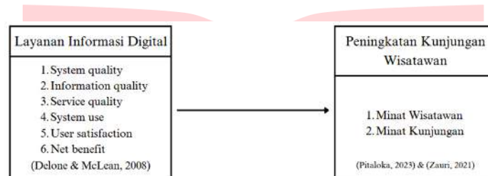
Gambar 1. Kerangka Pemikiran
