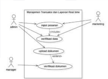
Gambar 4.4 Use Case Diagram Sumber : Data Diolah Peneliti
