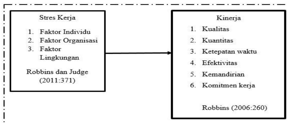
Gambar 2.2 Kerangka Pemikiran
