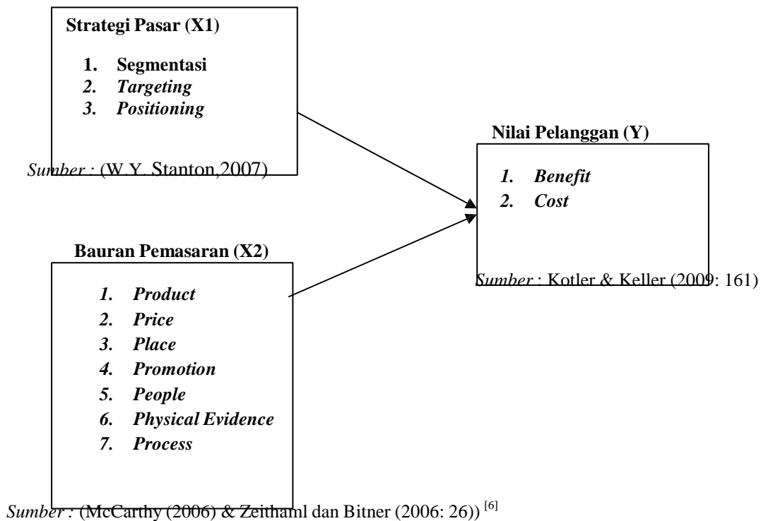
Gambar 2.1 Kerangka Pemikiran
