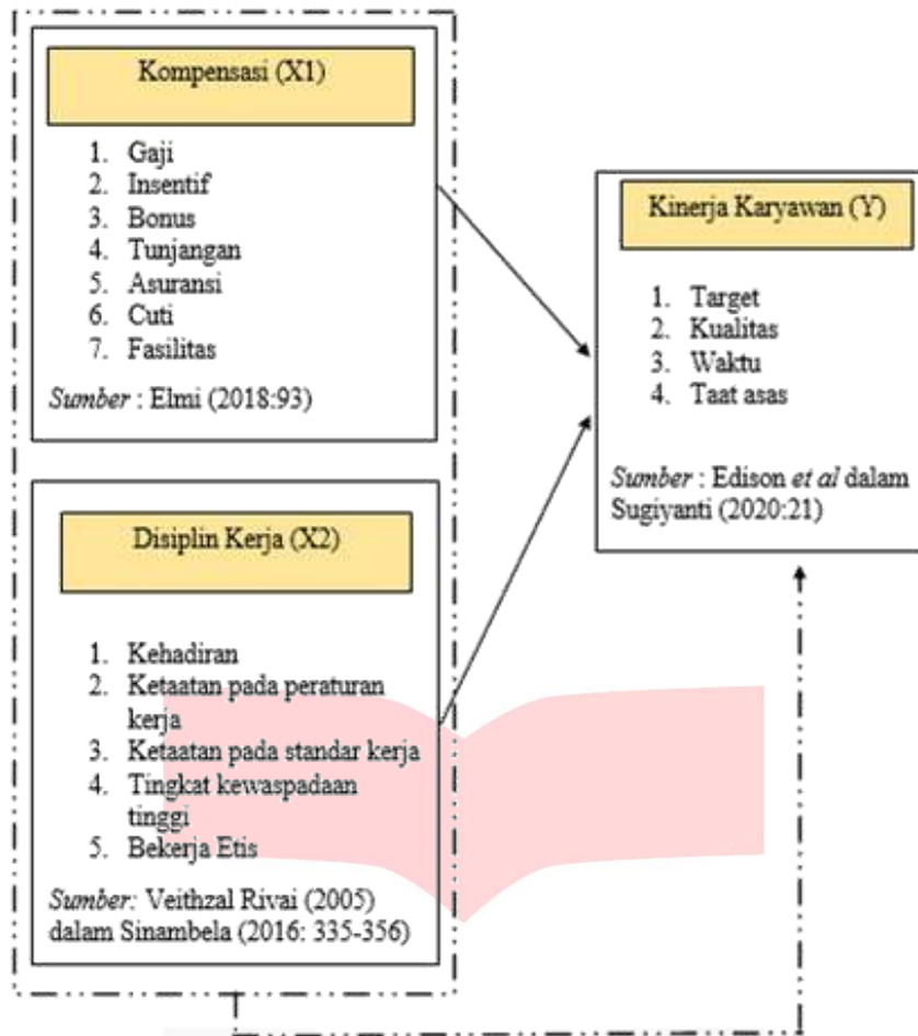
Gambar 2.1 Kerangka Pemikiran
