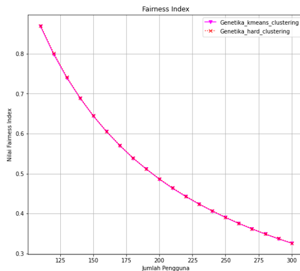
GAMBAR 6 GRAFIK FAIRNESS
