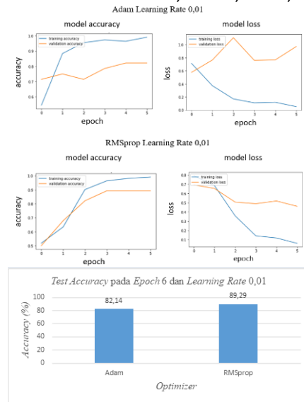
GAMBAR 7 TRAINING DAN TESTING & TEST ACCURACY PADA EPOCH, LEARNING RATE 0,01
