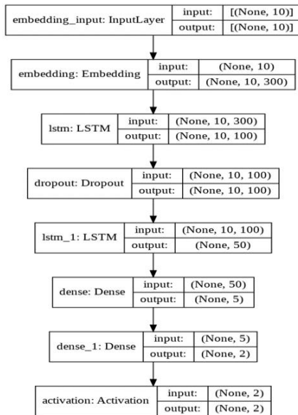
GAMBAR 3 ARSITEKTUR MODEL
