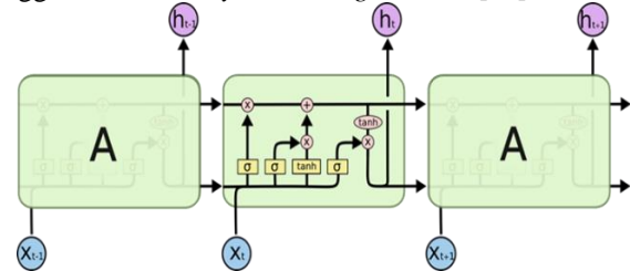
GAMBAR 1 ARSITEKTUR LSTM
