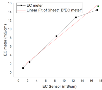
GAMBAR 12 PENGUJIAN SENSOR EC
