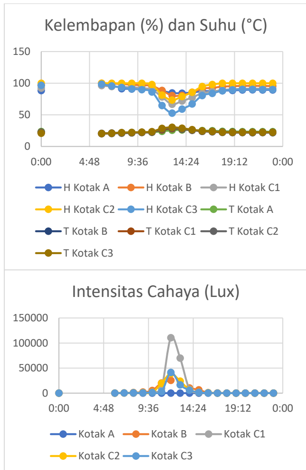
GAMBAR 15 GRAFIK KELEMBAPAN, SUHU, DAN INTENSITAS CAHAYA
