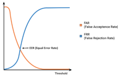
GAMBAR 5. KURVA RELASI ANTARA FAR, FRR, DAN EER
