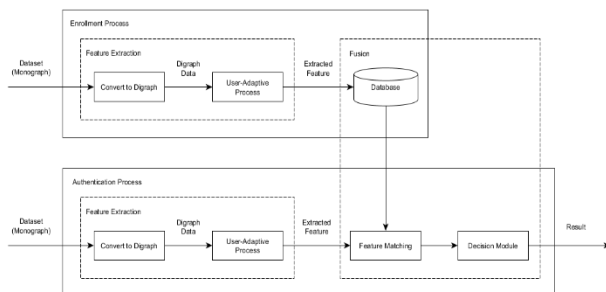
GAMBAR 6. SISTEM AUTENTIKASI DENGAN FITUR USER-ADAPTIVE DAN MAHALANOBIS DISTANCE
