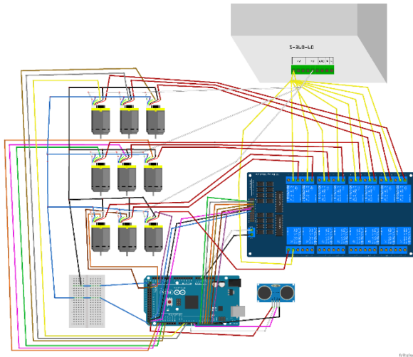
GAMBAR 2 SKEMATIK SISTEM
