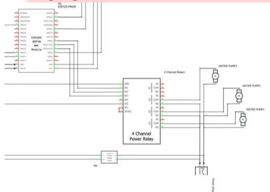
GAMBAR 2.4 Skematik pompa isi, kuras, dan sirkulasi
